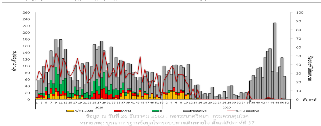
รูปที่ 1 จำนวนตัวอย่างที่ส่งตรวจของเชื้อไวรัสไข้หวัดใหญ่ 3 โครงการ จำแนกตามผลการตรวจทางห้องปฏิบัติการ รายสัปดาห์ ตั้งแต่วันที่ 1 มกราคม 2562 ถึงวันที่ 26 ธันวาคม 2563
